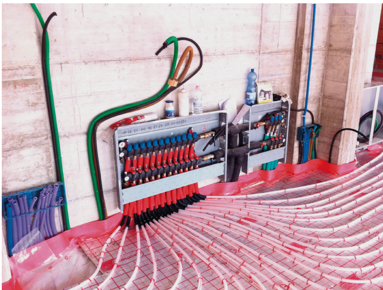
Figura 7.7 – Un collettore di distribuzione di un sistema radiante a pavimento prima del getto della caldina termica. Si faccia caso alla presenza della striscia di bordo, in EPDM o altro materiale finalizzato al conseguimento di una “vasca acustica”
